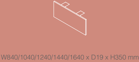
Modesty panel Séparateur frontal Faldón frontal Sichtschutzblende Painel frontal
